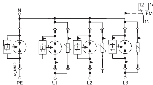
5SD7 444-1
