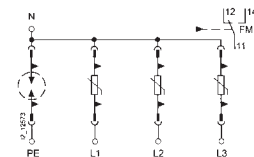
SSD7 464-0 kontaklı
