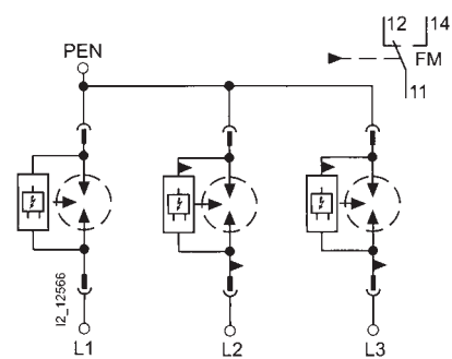
3-kutuplu 5SD7 413-1
