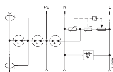
5SD7 435-5, 5SD7 435-7
