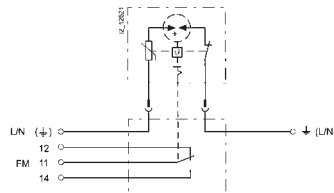
SSD7 461-0 kontaklı
