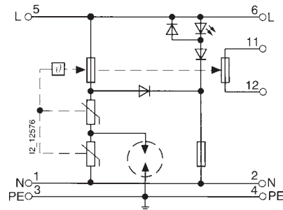
2-kutuplu 5SD7 432-
