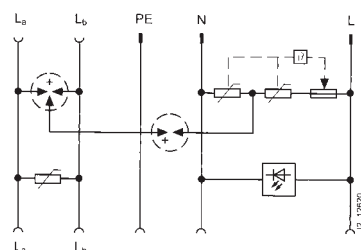
5SD7 435-6
