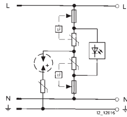
5SD7 435-0
