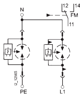
2-kutuplu 5SD7 412-1
