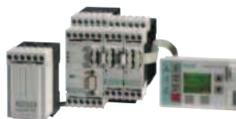
SIMOCODE PRO V
