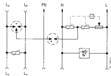
5SD7 435-2
