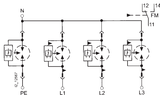
4-kutuplu 5SD7 414-1
